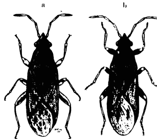
Abb. 3. Heterogaster canariensis n. sp. (a), H. artemisiae (Schill.) (b).
