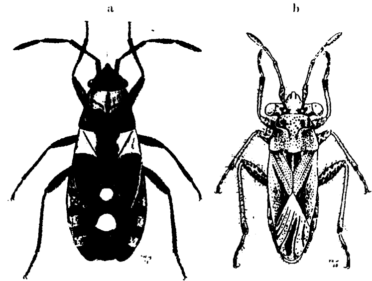
Abb. 2. Melanocoryphus albomaculata n. sp. ♂ (a), Henestaris wagneri n. sp. ♀ (b).
