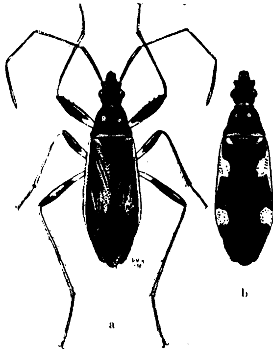
Abb. 5. a: Nouthieria pieltaini Menor, b: var. fernandesi Lindb.
