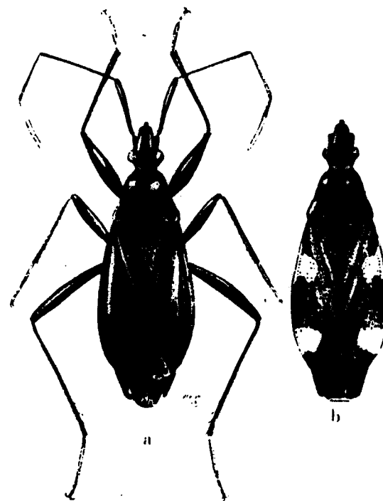
Abb. 4. Noualhieria quadripunctata (Brullé) var. coracipennis Put. (a), N. quadripunctata (Brullé) (b).
