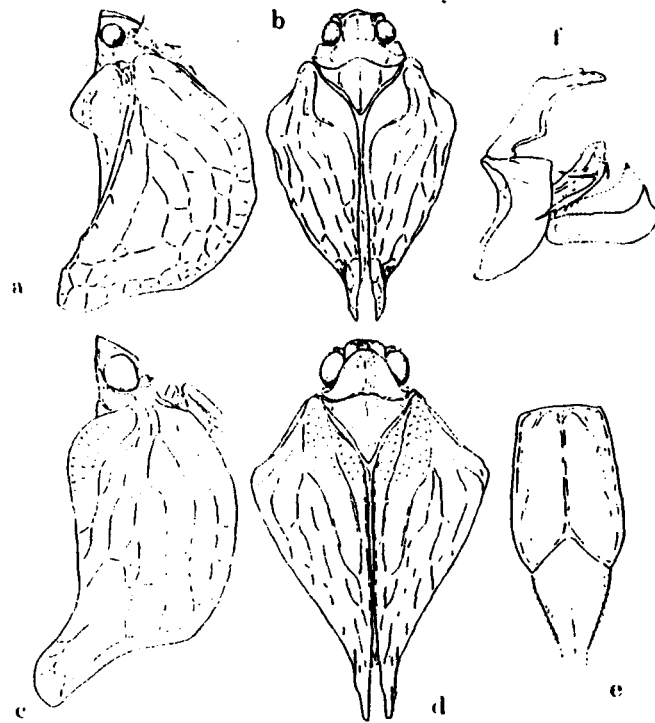
Abb. 7. Cyphopterum palmense n. sp. ♀: a. von der Seite, b. von oben. — C. moralesi n. sp. ♂: c. von der Seite, d. von oben, e. Stirn, f. Hinterleibsspitze mit männlichen Genitalien.
