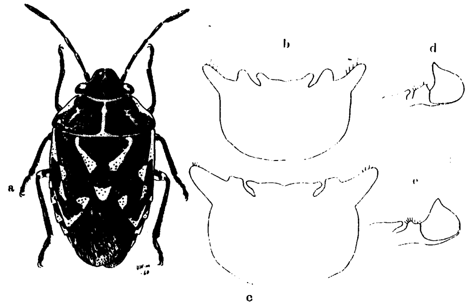
Abb. 1. Eurytoma lundbladi n. sp. ♂: a. Habitusbild, b. Genitalsegment von oben, d. Hinterecken desselben von hinten. — E. oleraceum (L.): c. Genitalsegment von oben, e. Hinterecken desselben von hinten.
